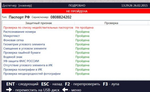
Окно программы с полным отчетом анализа документа
